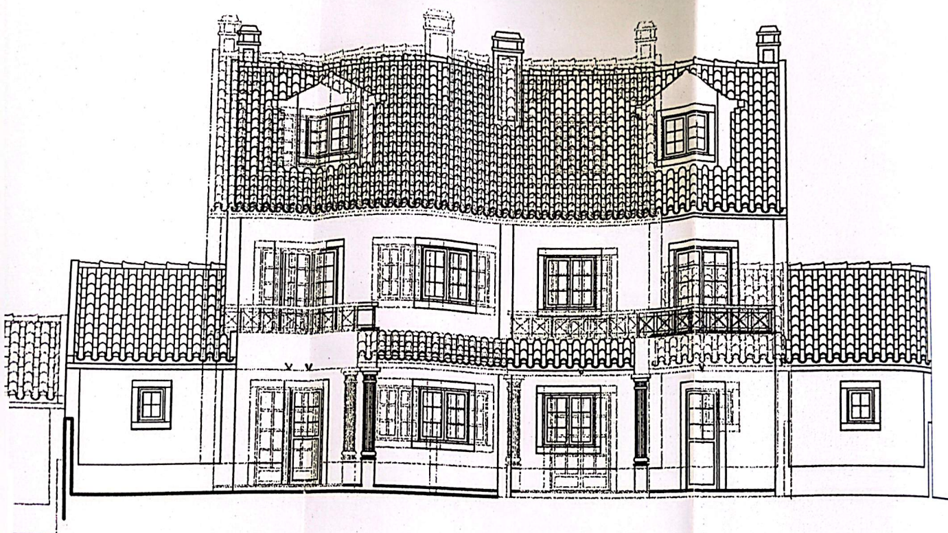
ALÇADO POSTERIOR
