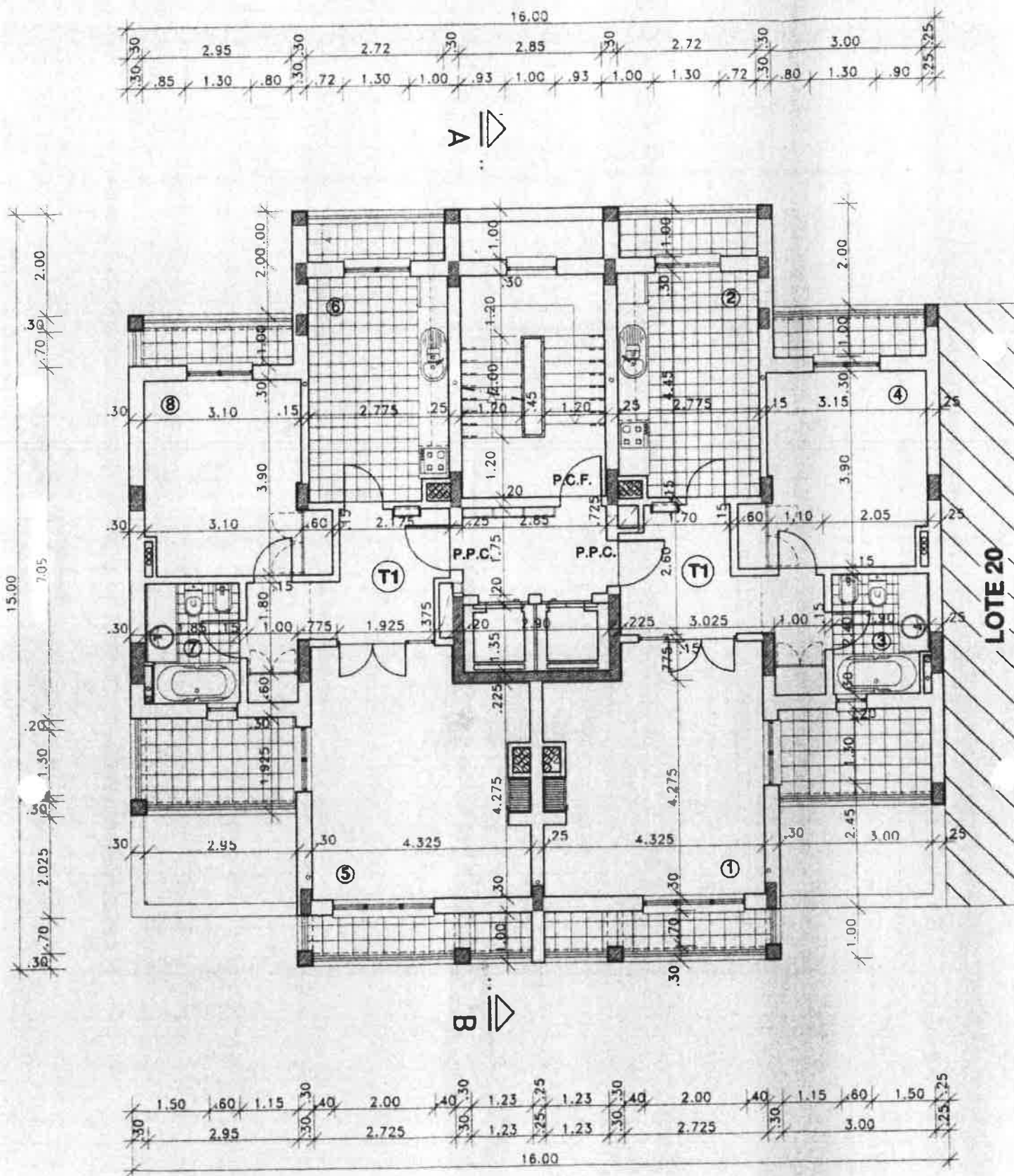
PLANTA DO 5º ANDAR
