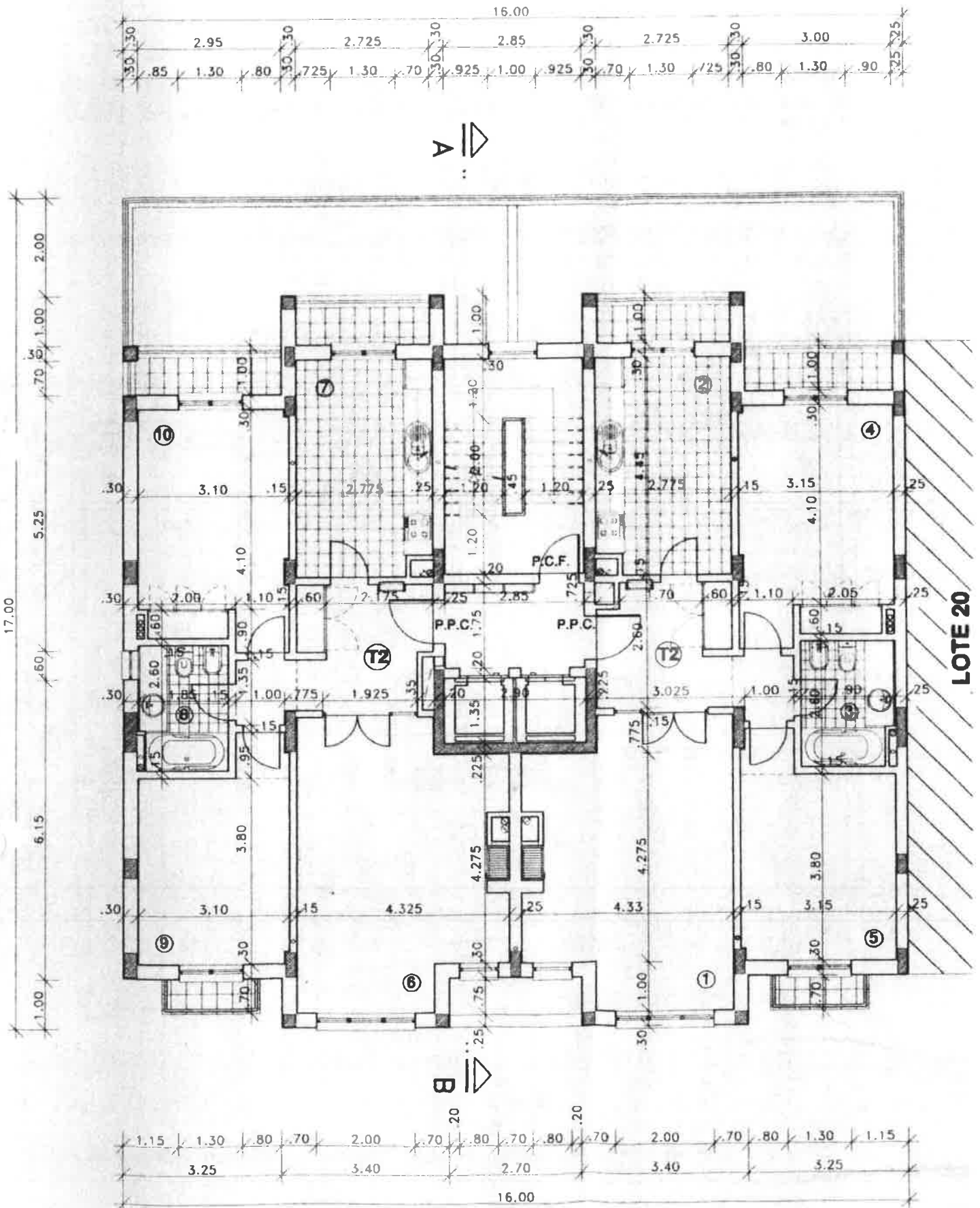
PLANTA DO 1º ANDAR
