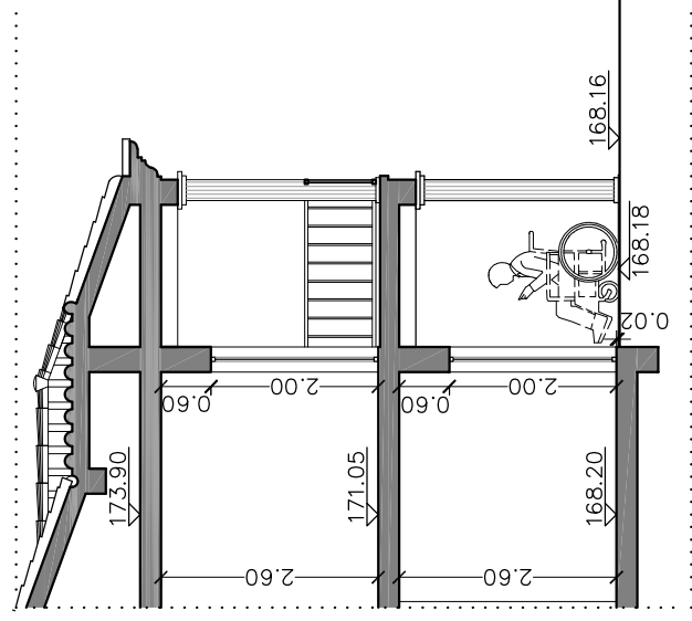
Corte 1/1' - Percurso Acessível Escala 1/100
