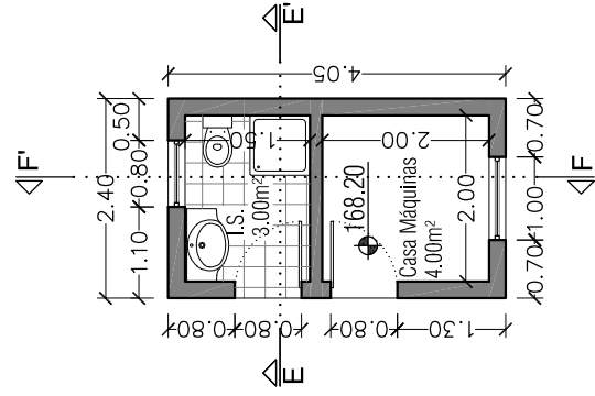
Planta do Piso 1
