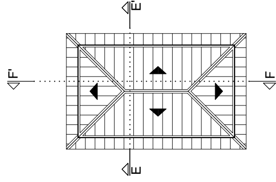
Planta da Cobertura
