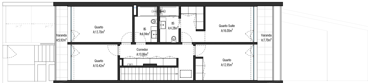
Planta Piso 1
