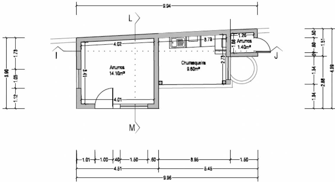
Planta do Piso Térreo
