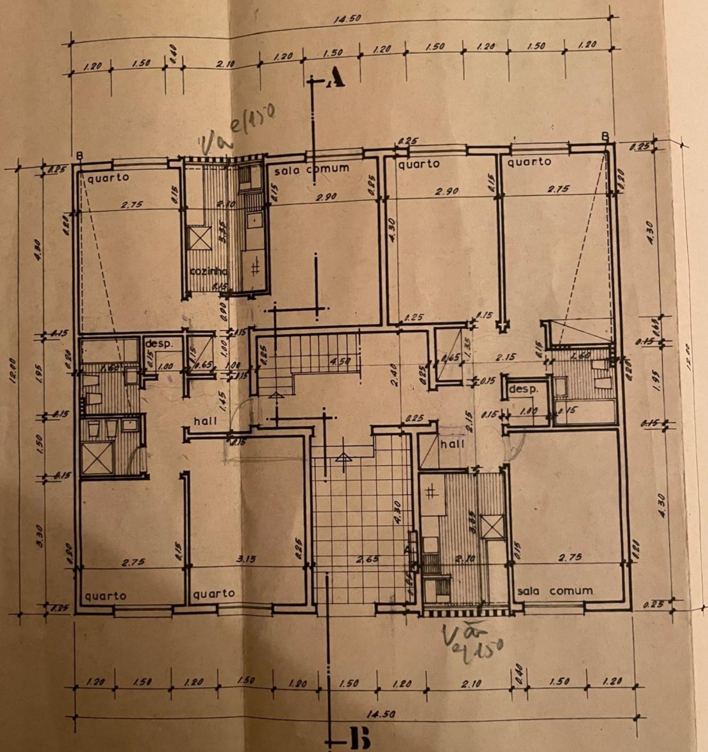
planta do nível da entrada
